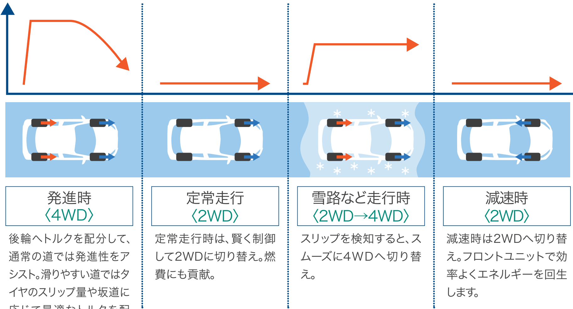
前後輪トルク配分イメージ
